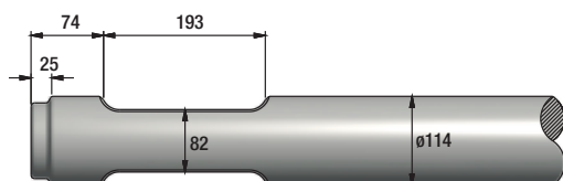
FIGURE 150 ITALDEM GK 1050
