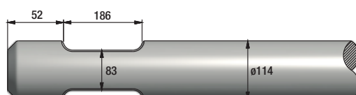
FIGURE 151 ITALDEM GK 1350
